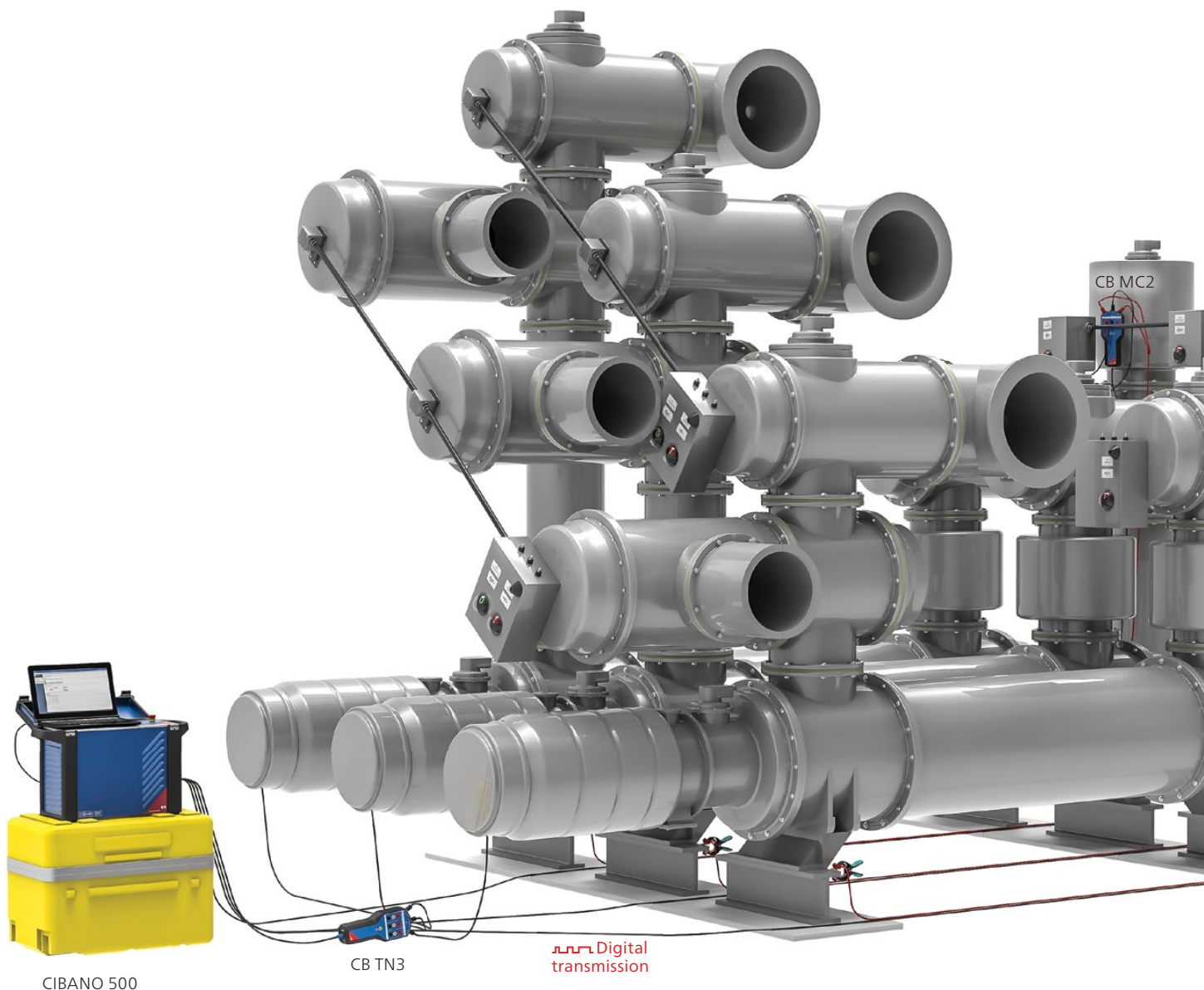
CIBANO 500
